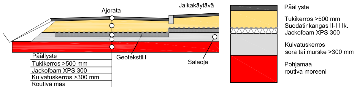
Routaeristetty katupoikkileikkaus
