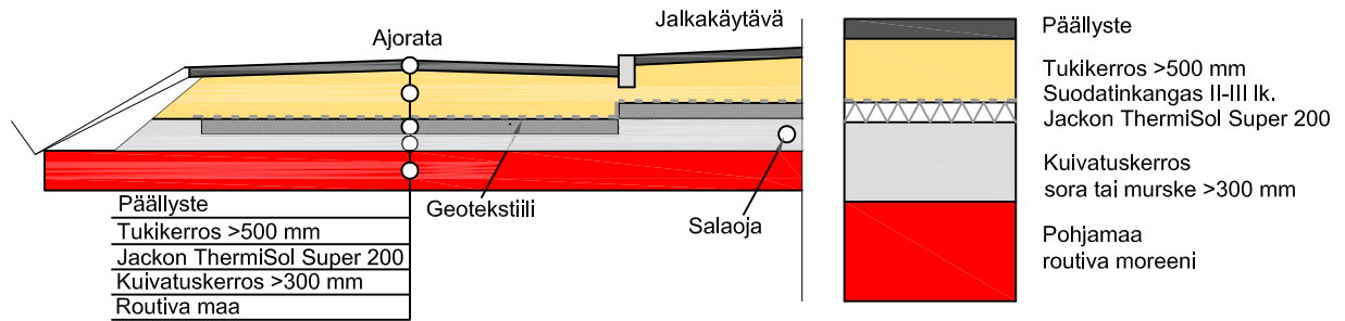
Routaeristetty katupoikkileikkaus
